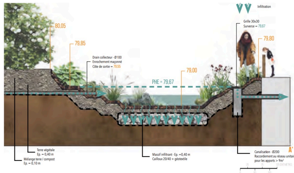
Coupe du bassin d'infiltration de la cours de l'école maternelle de Saint-Cloud :
